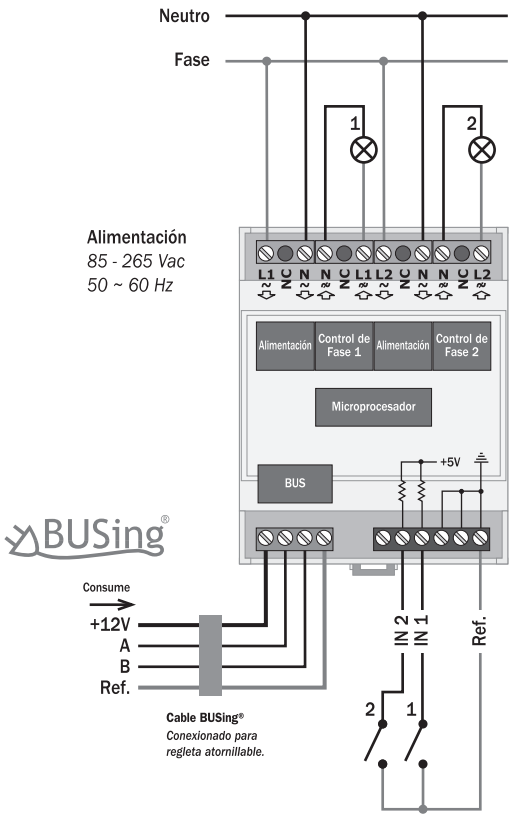
Cableado de las entradas RU2S200 Todas las entradas son SELV. Están referidas internamente a 5 V y se activan al conectarlas a masa.
